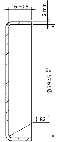
Section A-A
