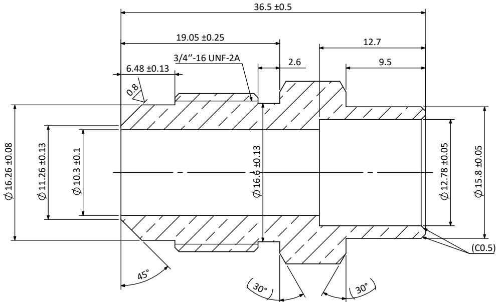
Section A-A
